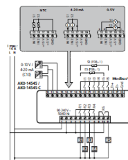
АКО-14545 /АКО-14545-С
